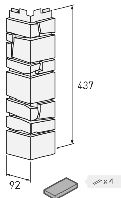
FS.252 финишный профиль
