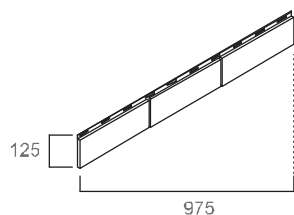
SC.LC цокольный профиль Solid Cube
