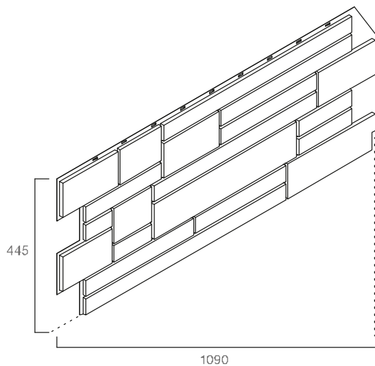
SC.LC цокольный профиль Solid Cube
